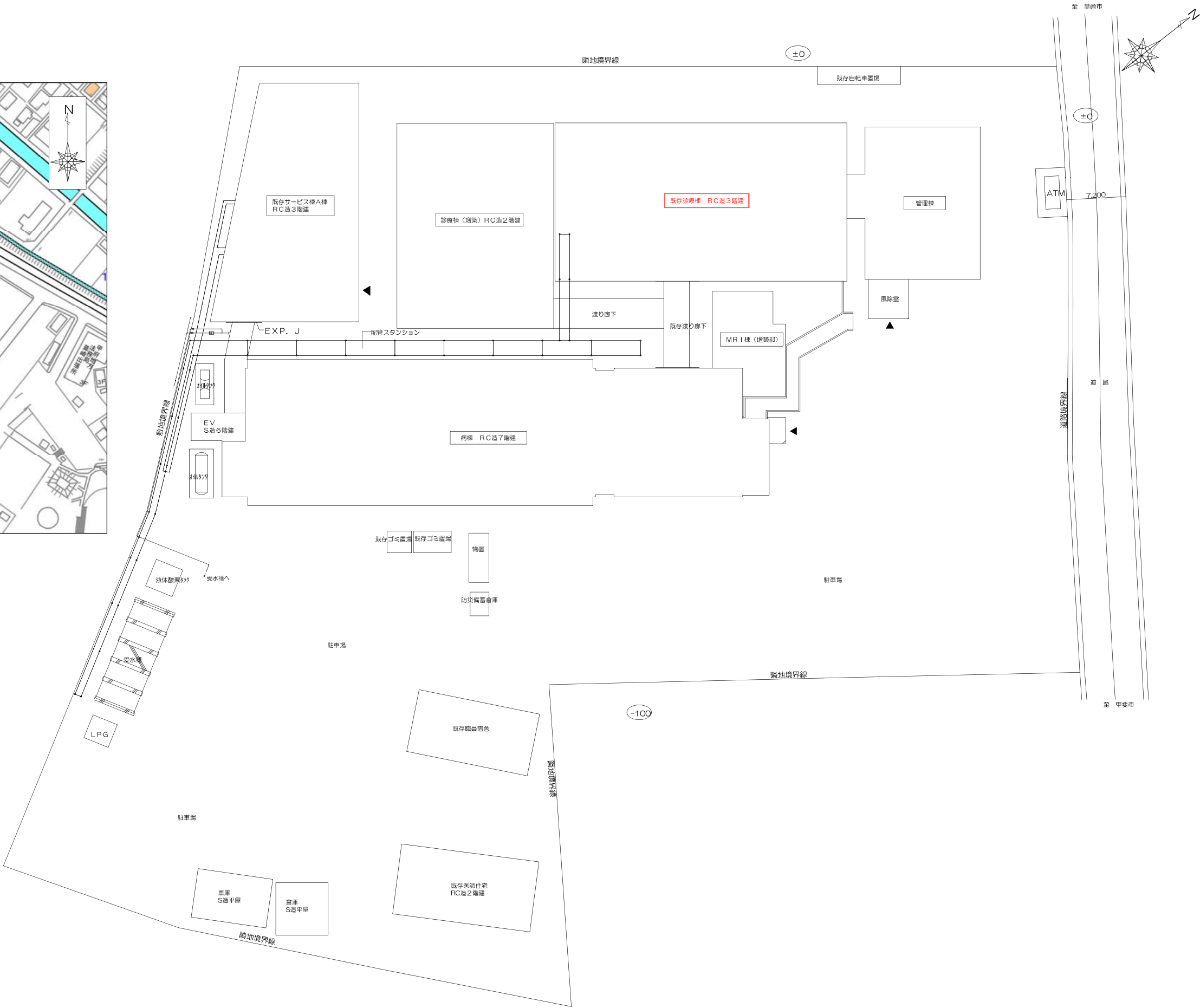
配置図 1/500 ※赤字：工事対象箇所
