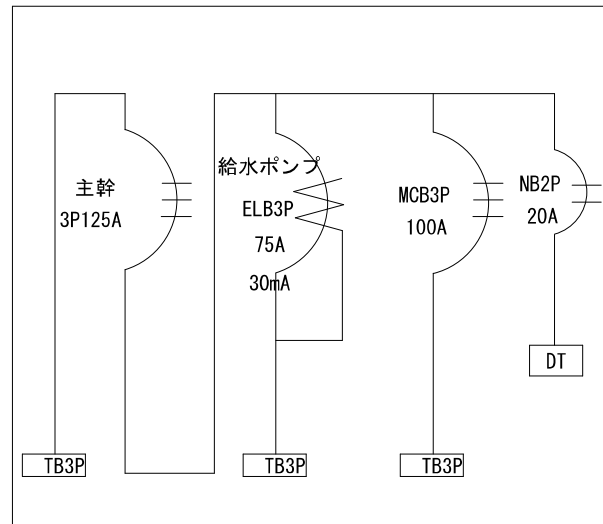
動力盤
