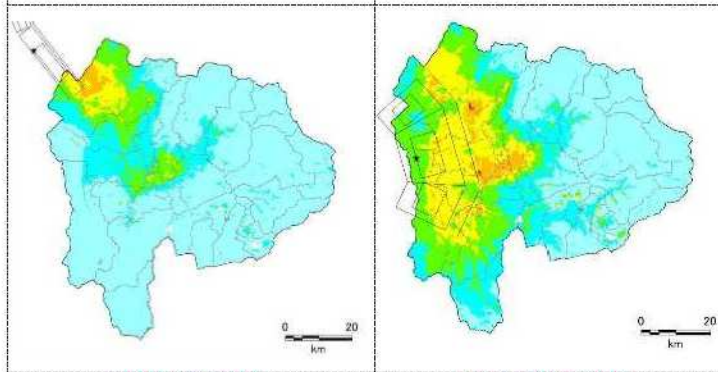
図6 地表震度分布 糸魚川-静岡構造線 中南部区間
